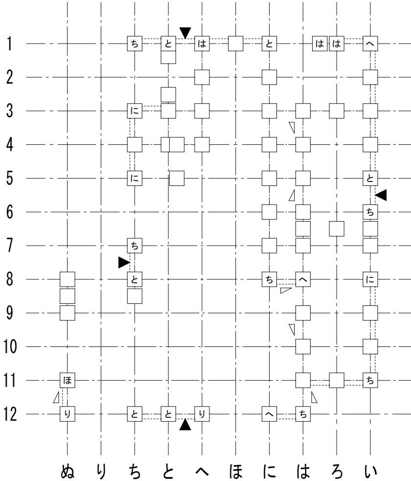
1 階柱壁伏図
