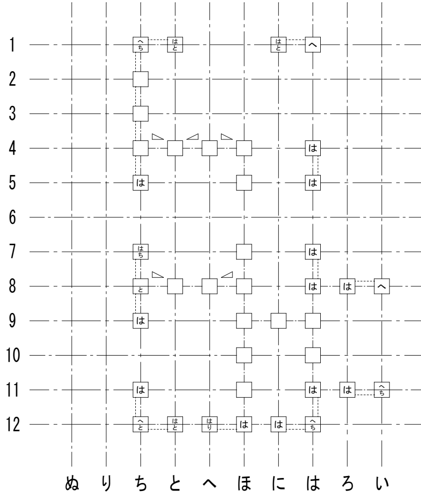
2 階柱壁伏図
